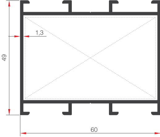
KASA PROFİLİ
