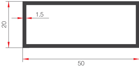
6594 AĞIRLIK (kg/m) / WEIGHT 545
