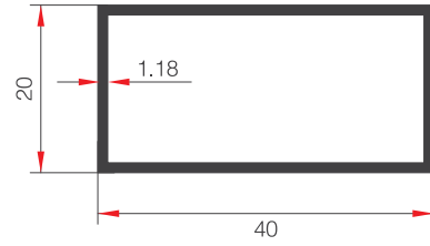
37689 AĞIRLIK (kg/m) / WEIGHT 368.6
